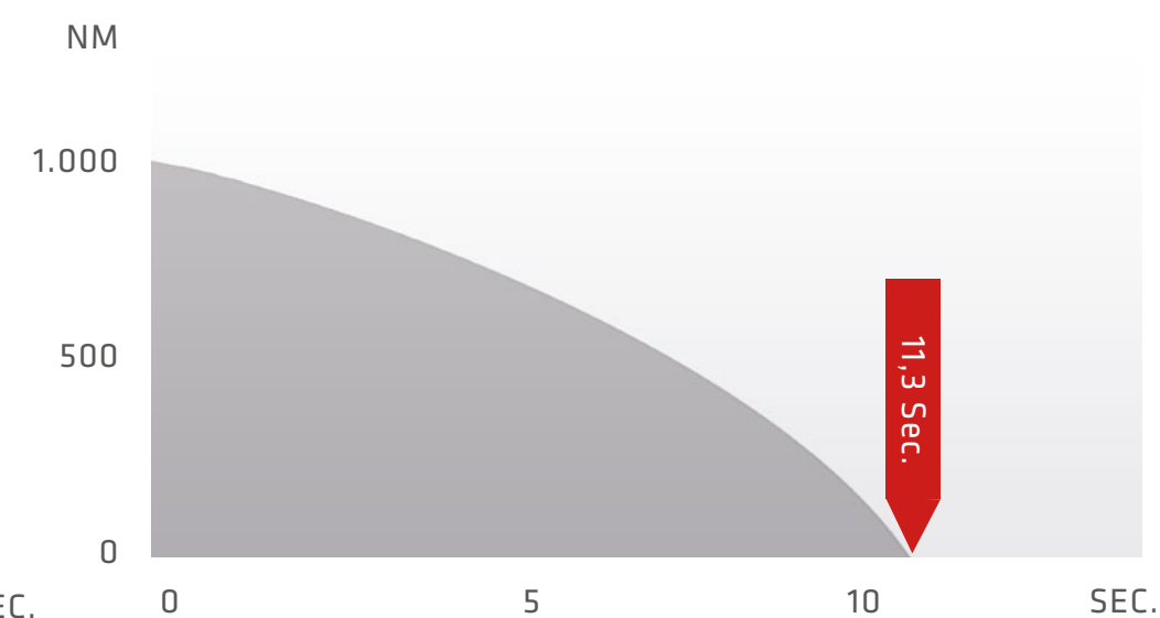
Desserrage : courbe de couple de la SW C5144
