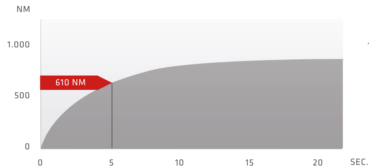
Serrage (position 2) : courbe de couple de la SW C5144
